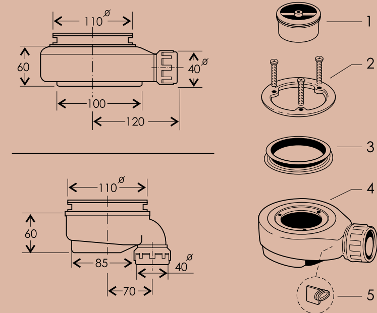
Válvula Doccia VH y VV
